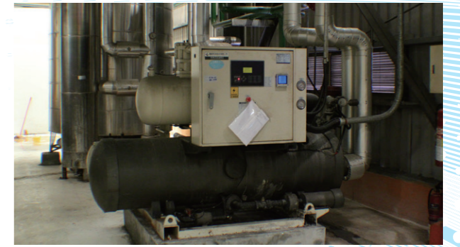
新增冰水機熱泵取代蒸氣
