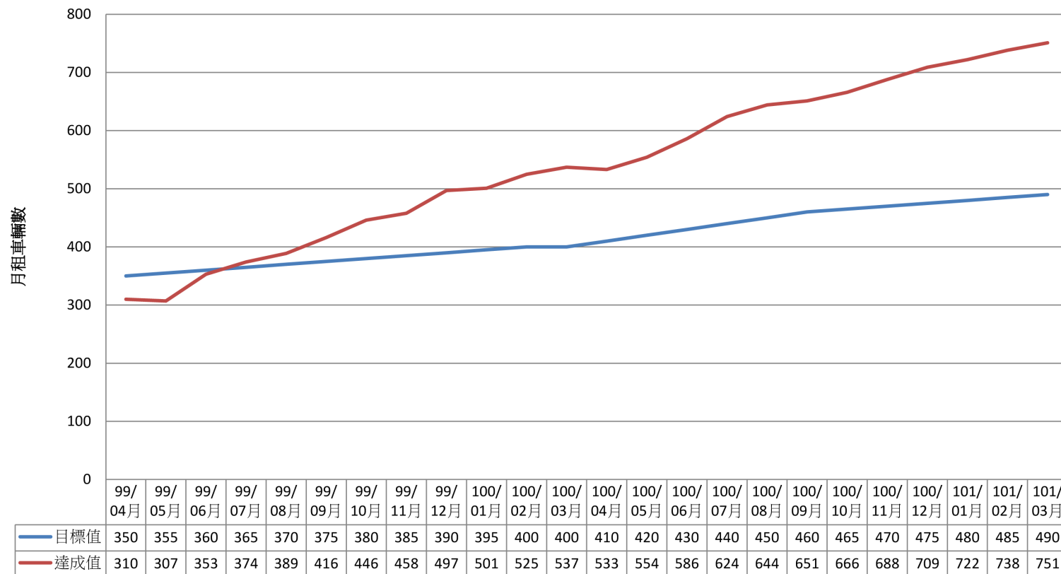
第1月-24月月租車營業達成值與計畫書目標值比較表
